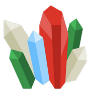
Minerals
